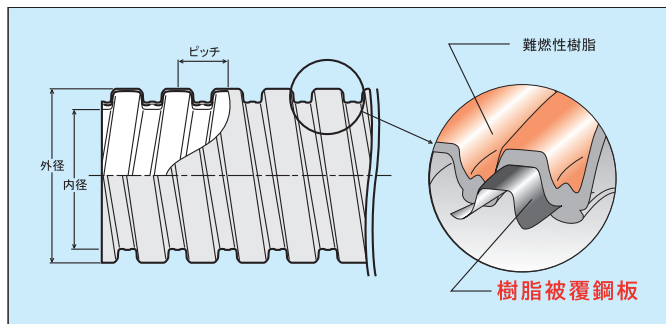
構造図
